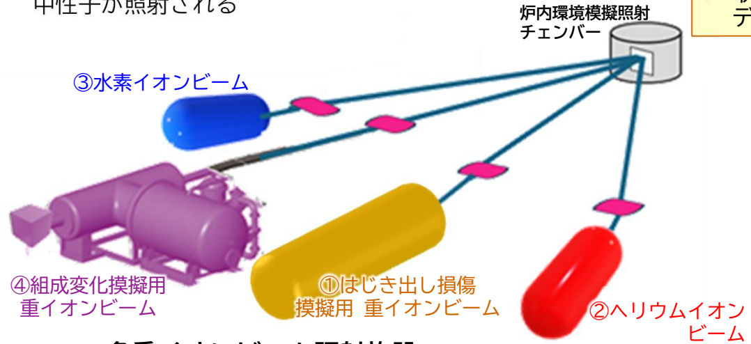
多重イオンビーム照射施設 (4MV、3MVタンデム加速器、2MVシングル加速器x2 (計画))
