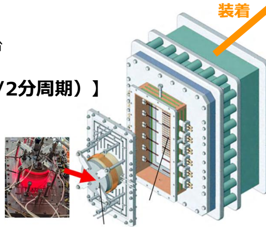
直流/高周波 ハイブリッド放電型 研究開発用 負イオン源 (~100 keV / 数A)
